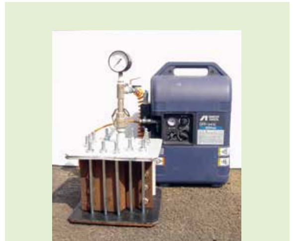
写真-13 試験装置全景
