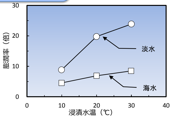
図1 浸漬水温と膨潤率
