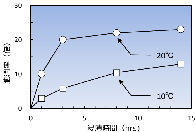
図2 浸漬時間と膨潤率
