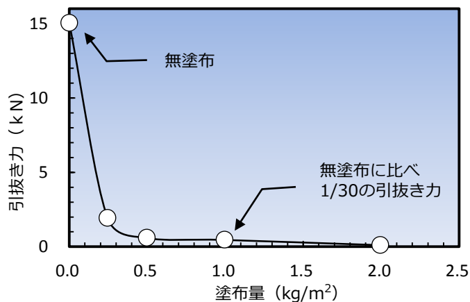
図4 ラブケミカ塗布量と引抜き力
