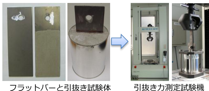
図3 模擬仮設杭の引抜き試験
