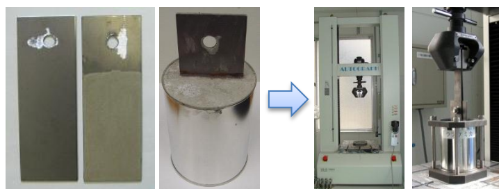
図3 模擬仮設杭の引抜き試験
